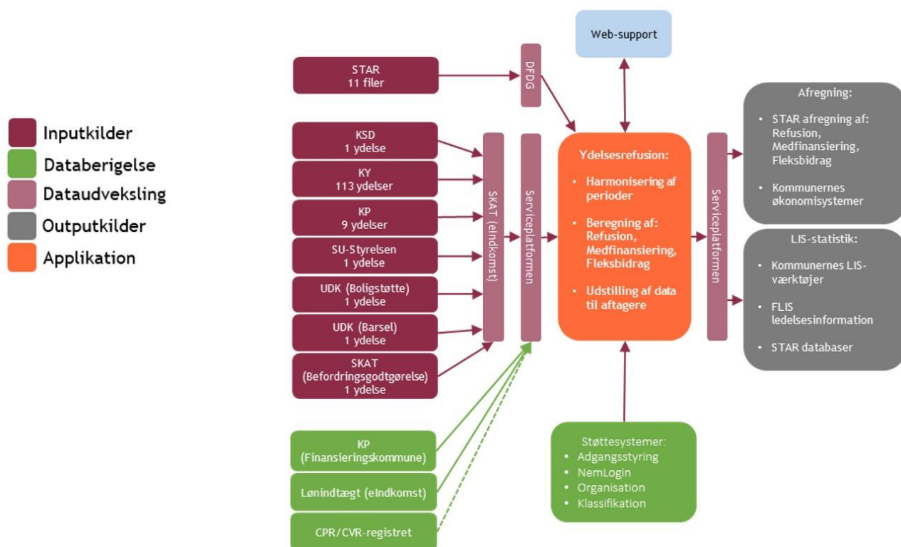
Figur 1: Ydelsesrefusion og snitflader til ind og uddatasystemer
